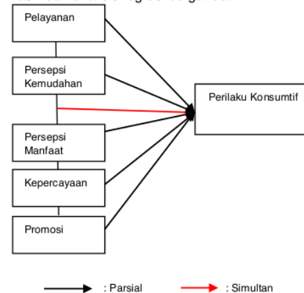
Gambar 1. Kerangka Berpikir
